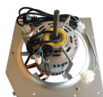
220516 FAN MOTOR 650W (80016072)
